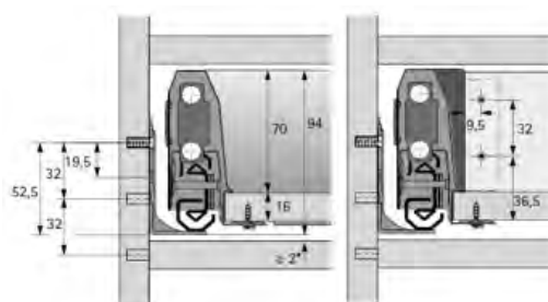
Posiciones de taladro, altura mínima montaje Drilling positions, minimum mounting height
