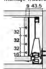
Montaje Trasero
