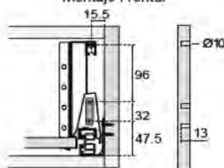
Montaje Frontal
