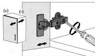
Ajuste de profundidad Depth adjustment
