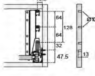
Montaje Frontal
