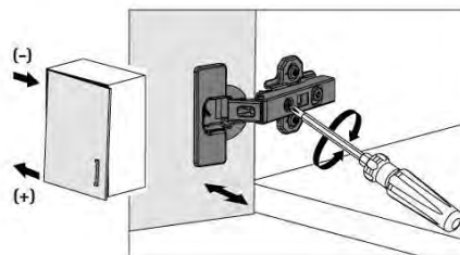
Ajuste de solapadura Side adjustment
