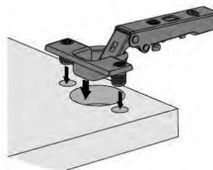
T43/TH-53 montaje directo T43/TH-53 press-in assembly
