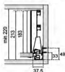
Montaje Mínimo Requerido
