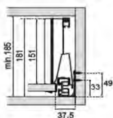
Montaje Mínimo Requerido
