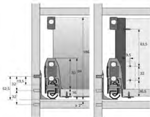
Posiciones de taladro, altura mínima montaje Drilling positions, minimum mounting height
