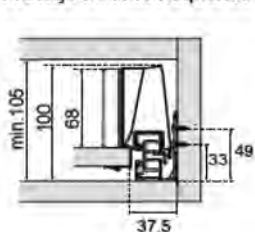
Montaje Mínimo Requerido
