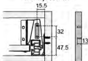
Montaje Frontal
